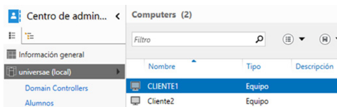
Imagen 54. Crear equipos 3.
