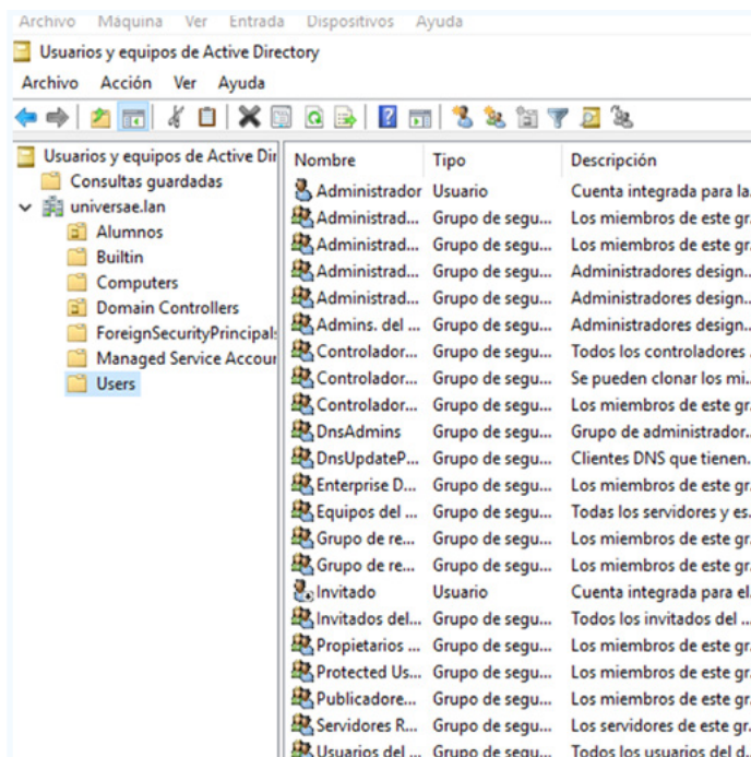
Imagen 1. Carpeta Users.
