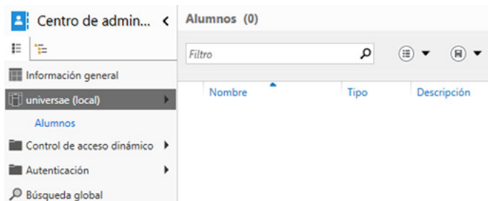
Imagen 48. Eliminar grupos 4.
