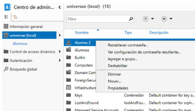
Imagen 14. Eliminar usuarios 1.
