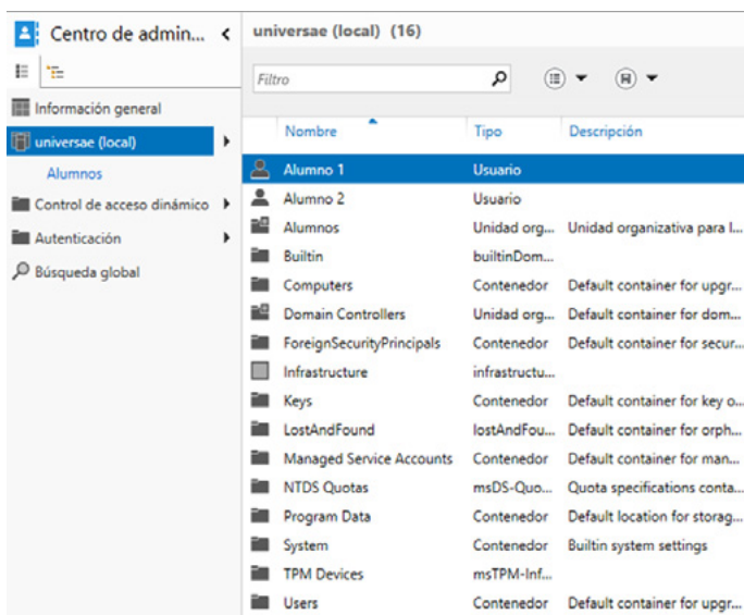
Imagen 49. Eliminar grupos 5.
